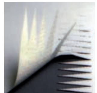
Endlosverbindungsarten, 1-lagiger Gurt, Einzelfinger bei 90°-Winkel
